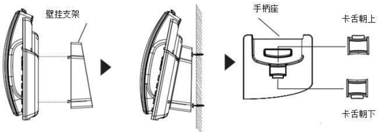
图 4: 壁挂安装
